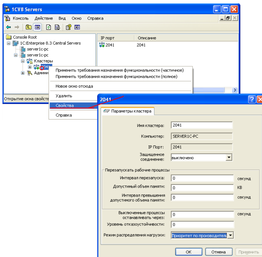
Рисунок 13. Просмотр и изменение свойств кластера
