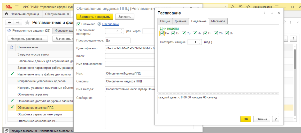
Рисунок 6. регламентные и фоновые задания
